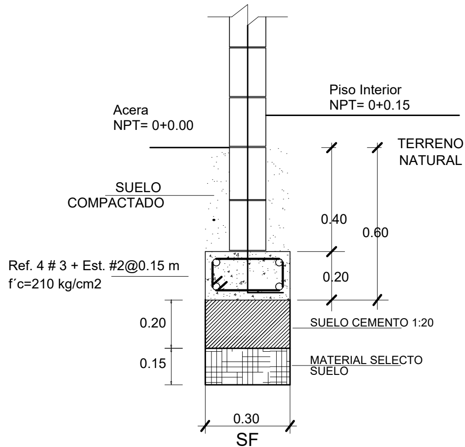
SOLERA DE FUNDACIONES ESC. 1:20
