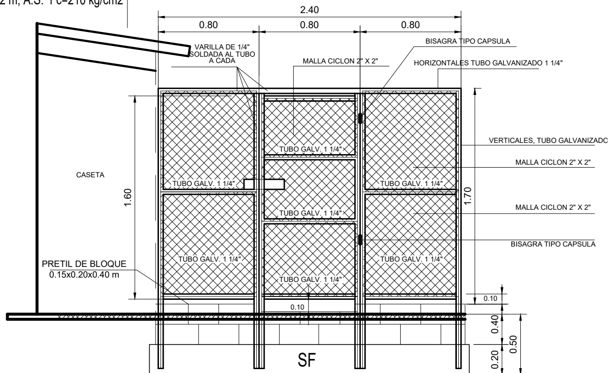
ELEVACION CERCO PERIMETRAL SIN ESCALA
